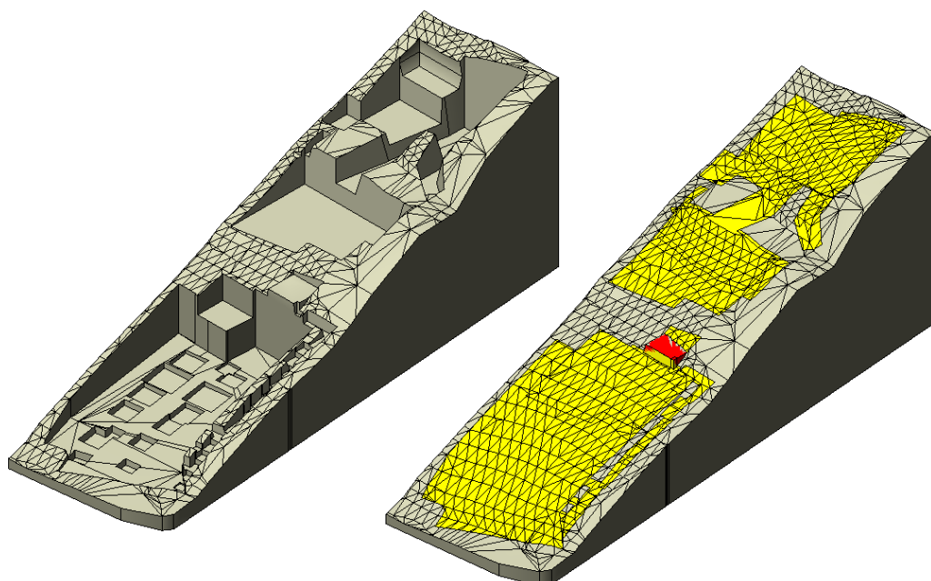
Interaktive Baugrube
