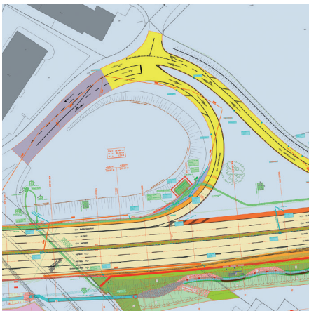
Projekt: Instandsetzung Autobahn A2 Stansstad-Beckenried, Büro: CES Bauingenieur AG
